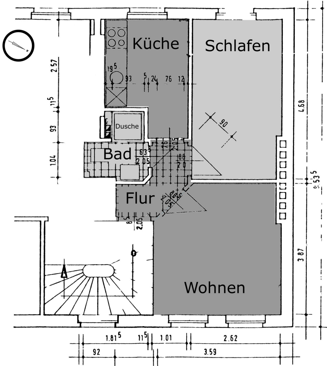
Grundriss Geibelstr. 37 - 3. Obergeschoss M 1:50
